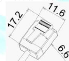
コネクター寸法図
