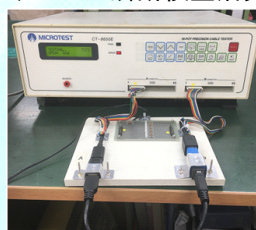
ケーブル瞬断検査治具
