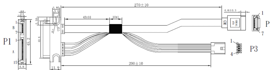
SATAデータケーブル
