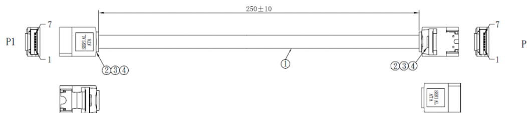
SATAデータケーブル
