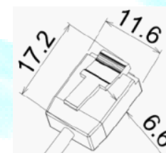
コネクタ寸法図
